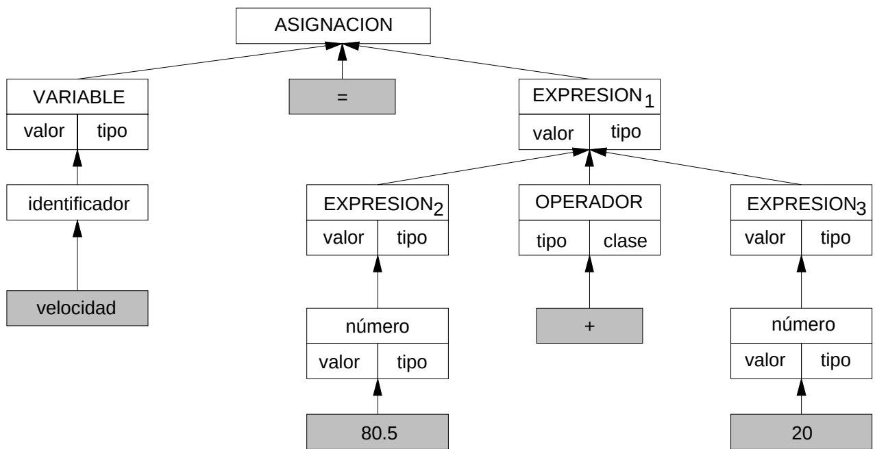
Figura 27: Arbol sintáctico con atributos
