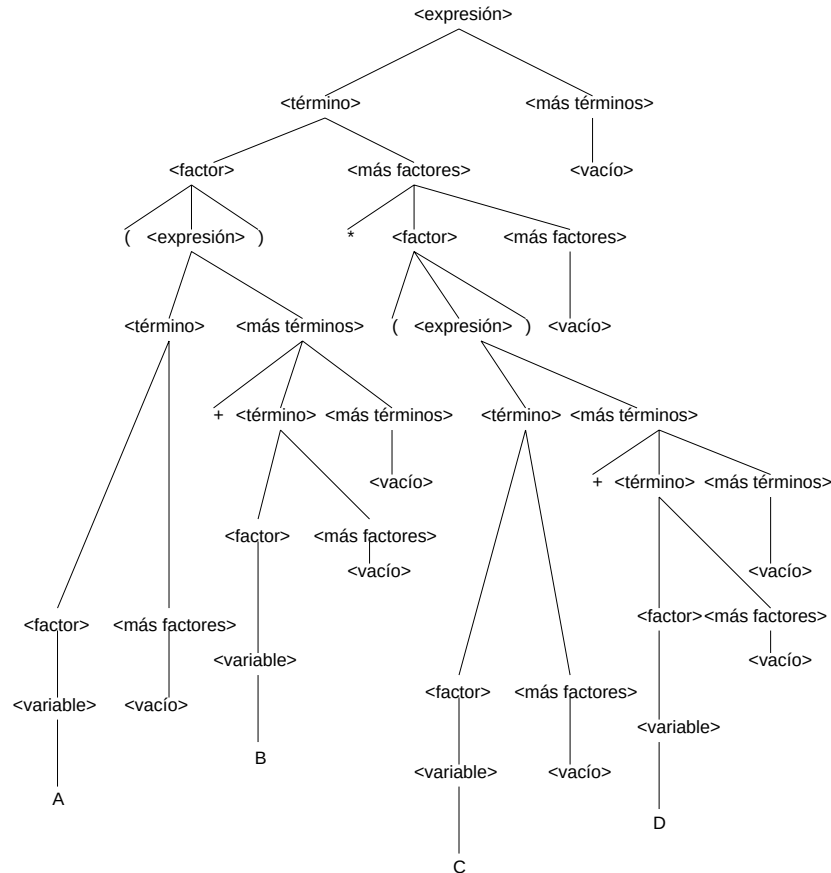
Fig. 29: Árbol sintáctico
