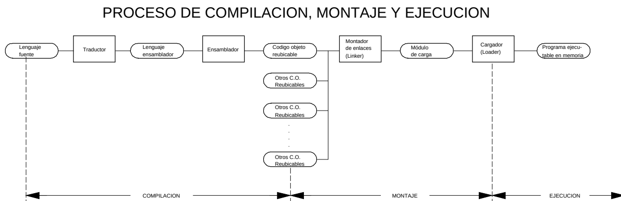
Fig. 8: Fases de compilación, montaje y ejecución
