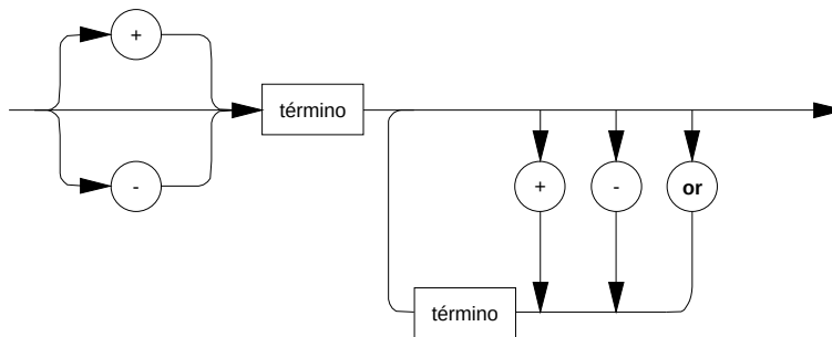
Expresión simple
